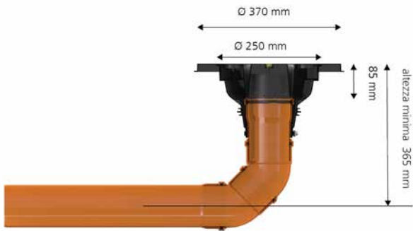
Misurazione del cono di raccordo AT110
