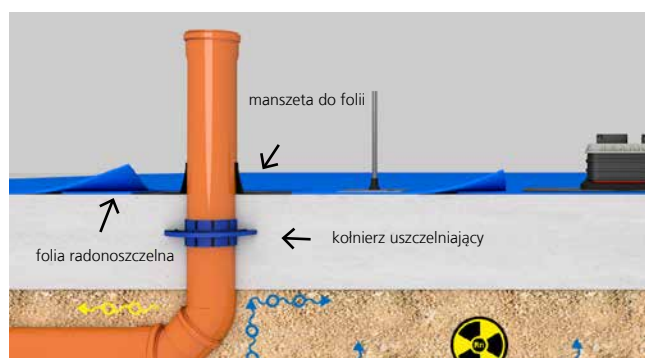
Uszczelnienie przewodów kanalizacyjnych za pomocą kołnierza uszczelniającego i przyłączeniu folii radonoszczelnej przez manszetę uszczelniającą.
