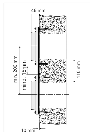
przekrój i wymiarowanie
