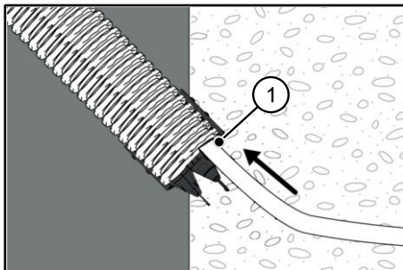
1 umgestülpte Tülle
