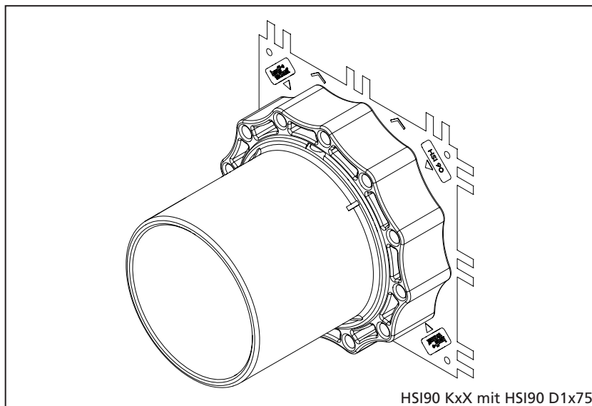
HSI90 KxX mit HSI90 D1x75
