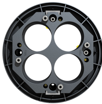
Mehrfach-Hausausführung ETGAR Außendichtelement
